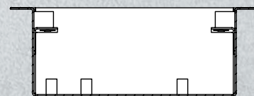
Boîtier de montage arrière (encastré)
